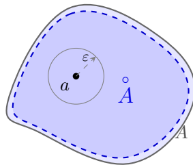
Point intérieur a et Intérieur \overset{\circ}{A} \exists \varepsilon > 0, B(a, \varepsilon) \subset A Plus grand ouvert contenu dans A
