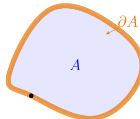
Frontière \partial A \partial A = \overline{A} \setminus \overset{\circ}{A} Séparation entre l'intérieur et l'extérieur
