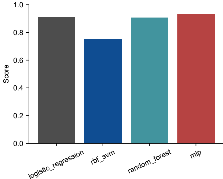
LOLO Macro-F1
