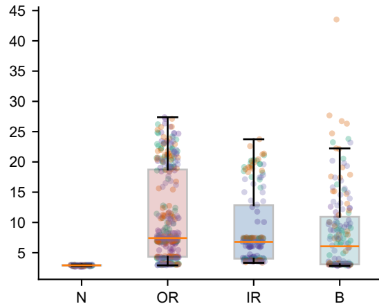
order_2_4
