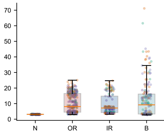
order_4_8
