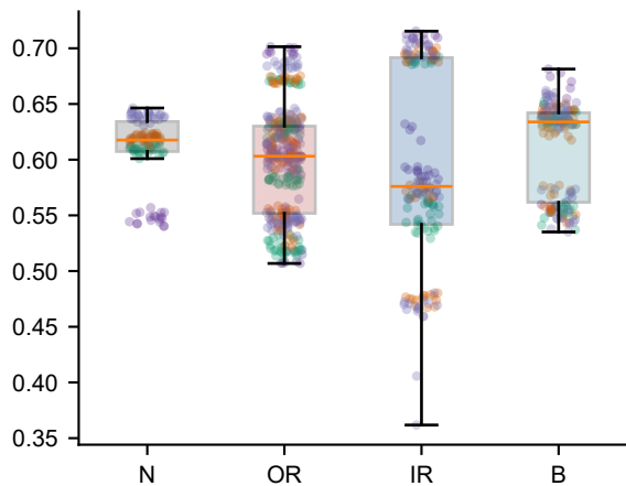
psd_entropy
