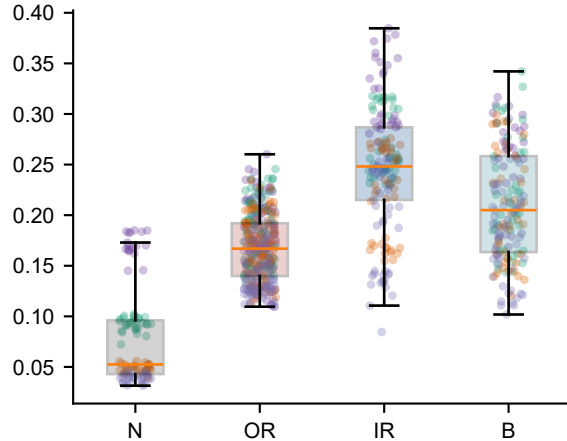
order_4_8
