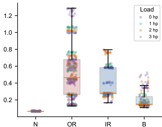
psd_entropy
