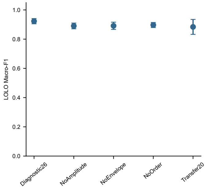
mlp
