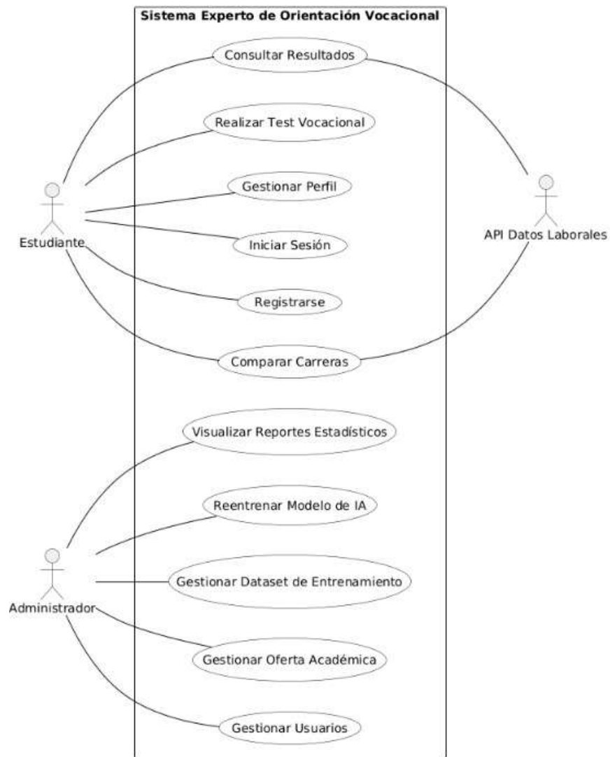
Ilustración 2. Diagrama de casos de uso
