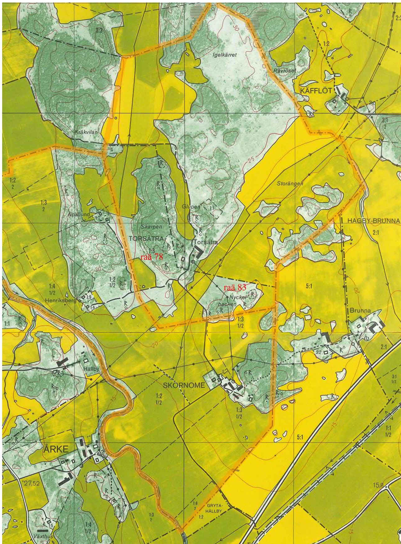
Figur 32. Torsätra i Hagby sn, Uppland, efter ek 11H5h och 11H6h. Gränser för Torsätra och Skornome efter gamla ekonomiska kartan (1860).
