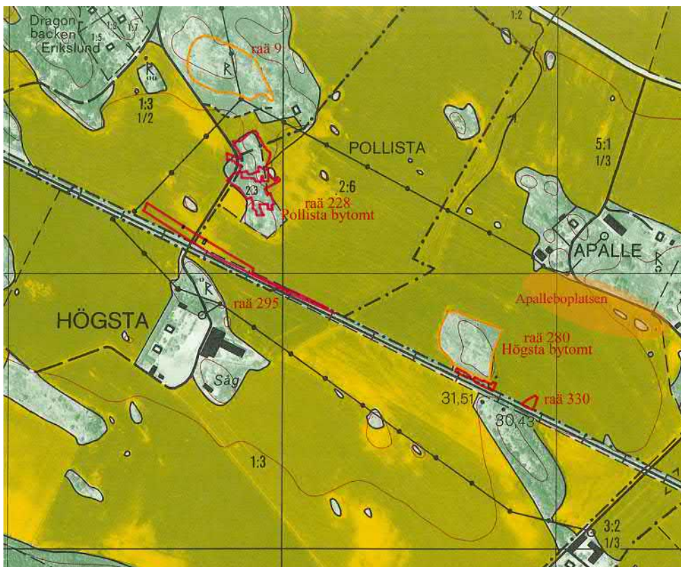
Figur 126. Bytomter, undersökningsytor [röda avgränsningar] och gravfält i Högsta och Pollista. Grundkarta ek 11H1i.
