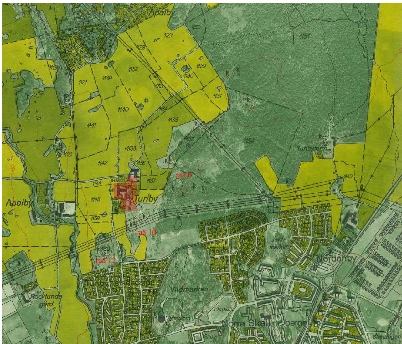
Figur 64. Undersökningsområdet vid Tunby ungefärligt markerat efter Annuswer & Karlsson 2003 fig. 1 s. 4. Grundkarta ek 1162i.
