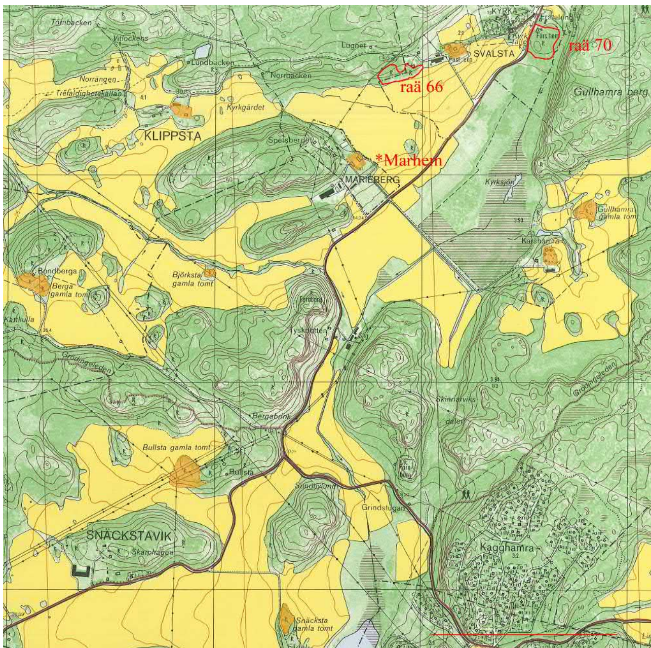
Figur 74. Marhemsbygden i Grödinge sn med äldre bytomter markerade. Grundkarta gula kartan 10I:01.
