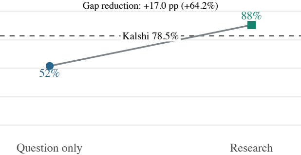
Gemini 3.1 Pro
