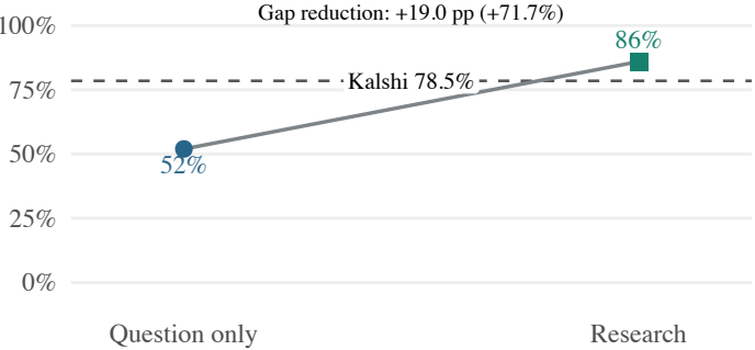
GPT-6 Astra
