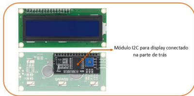
Figura 4: Display LCD 16 \times 2 e um adaptador LCD I2C.
