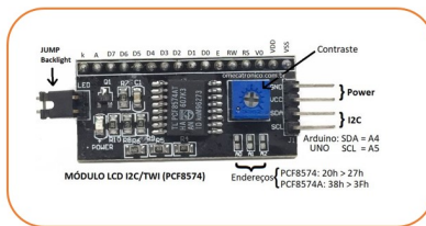
Figura 6: Pinagem do módulo I2C.
