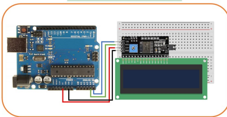
Figura 7: Pinagem do display I2C no Arduino.
