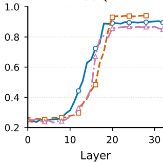
SciQ
