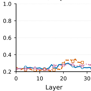
MathQA
