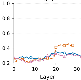
LogiQA
