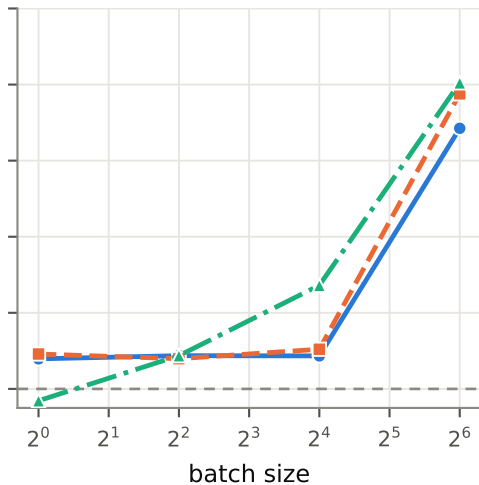
b 3BPA, 27 atoms
