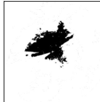
U-Net
