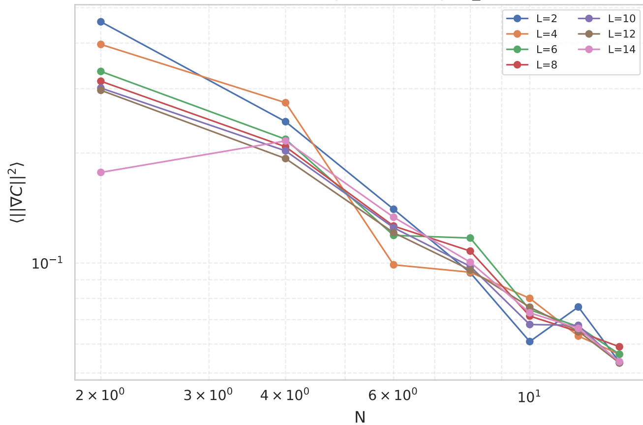
AT16 Heisenberg: Phase II (sigma_crit)
