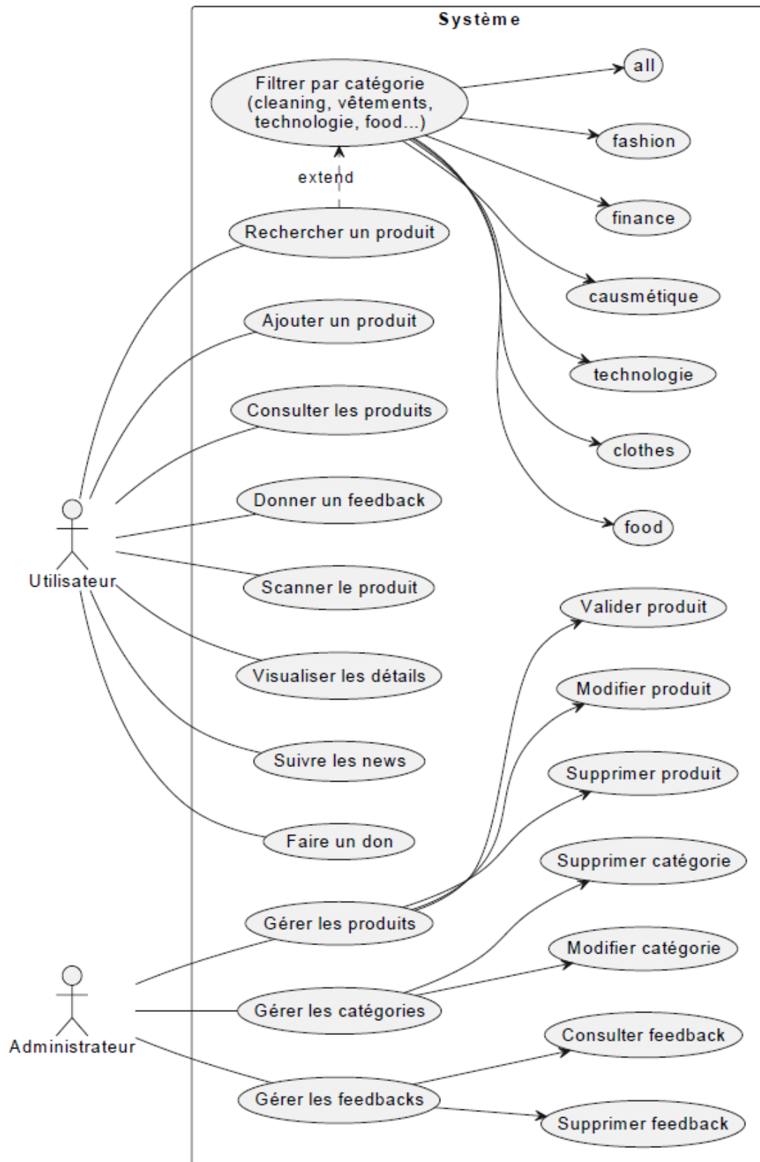
FIGURE 2.2 – Diagramme des cas d'utilisation
