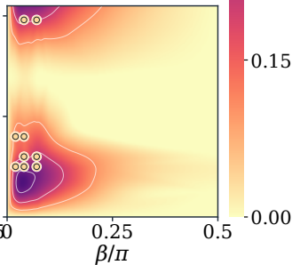
(d) dephasing
