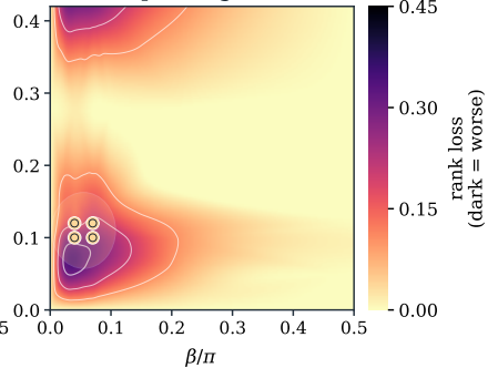
(d) dephasing channel
