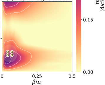
(d) dephasing channel
