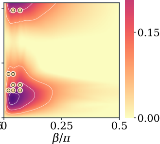
(d) dephasing
