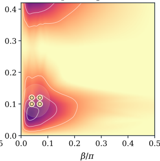
(d) dephasing channel
