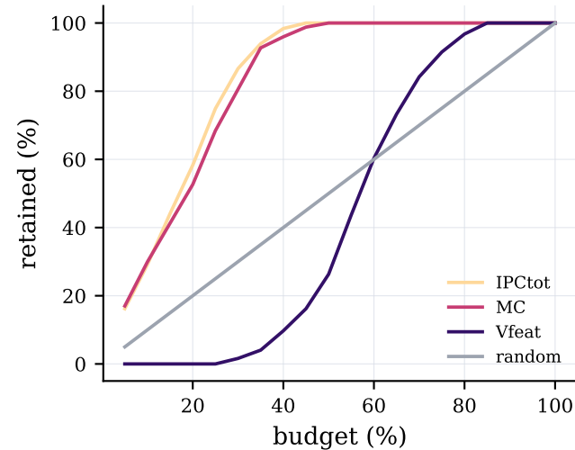
(d) screening retention
