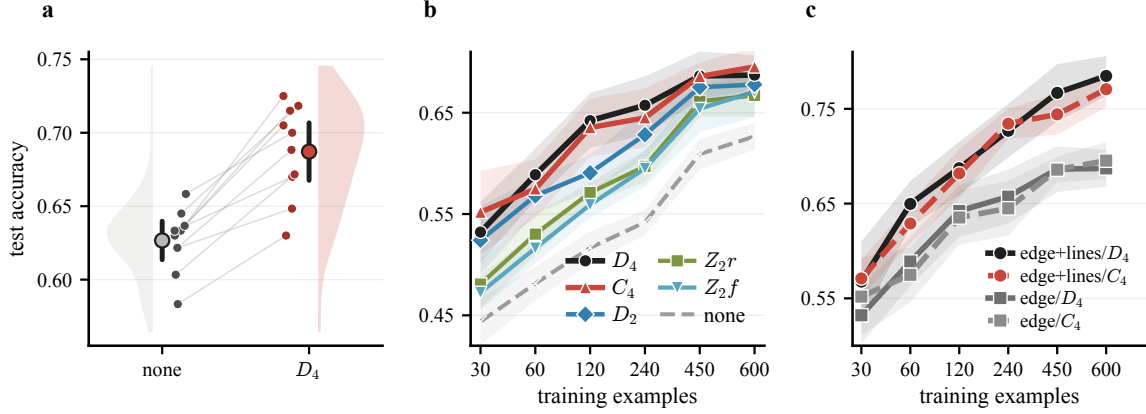
Abbildung 2: Hauptergebnisse aus dem finalen 10-Seed-Protokoll. Links: Reproduktion des Meyer-artigen Effekts, D_4 schlägt keine Symmetrie. Mitte: Untergruppen-Sweep über Trainingsgrößen 30 bis 600; C_4 folgt D_4 sehr eng. Rechts: Edge-Ansatz und Edge-plus-Line-Erweiterung über dieselbe Trainingsgrößenachse; die Winning-Line-Gates verbessern die Accuracy deutlich.
