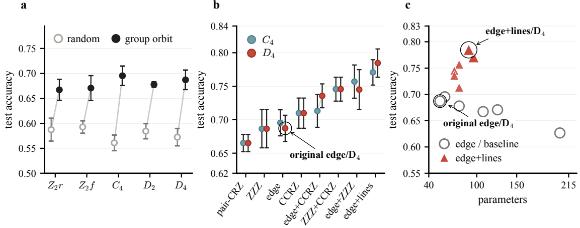
Abbildung 3: Controls und Ablationen aus dem finalen 10-Seed-Protokoll. Links: Parameter-matched random sharing schlägt group-orbit sharing nicht. Mitte: Ablation der Line-Gate-Familien bei 600 Trainingsbeispielen, aufsteigend nach mittlerer Leistung, mit dem markierten originalen Edge/ D_4 -Ansatz als Referenz. Rechts: Accuracy ist nicht allein durch Parameterzahl erklärbar; task-aligned equivariant geometry verschiebt das Modell in einen anderen Leistungsbereich.
