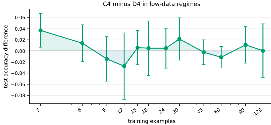
Abbildung 3: Low-Data-Zoom: Differenz der Test Accuracy zwischen C_4 und D_4 . Positive Werte bedeuten einen Vorteil für C_4 . Die Vorteile sind klein und nicht robust genug für einen Dominanz-claim, zeigen aber, dass partielle Symmetrie eine sinnvolle Modellwahlachse ist.
