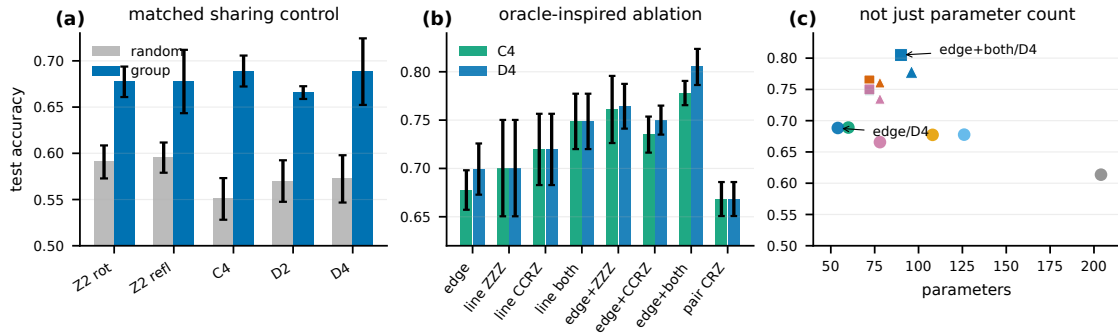
Abbildung 6: Controls und Ablationen. Links: Random sharing schlägt symmetry-aware sharing nicht. Mitte: Oracle-inspirierte Ablation bei 600 Trainingsbeispielen. Rechts: Accuracy ist nicht allein durch Parameterzahl erklärbar; task-aligned equivariant geometry verschiebt das Modell in einen anderen Leistungsbereich.
