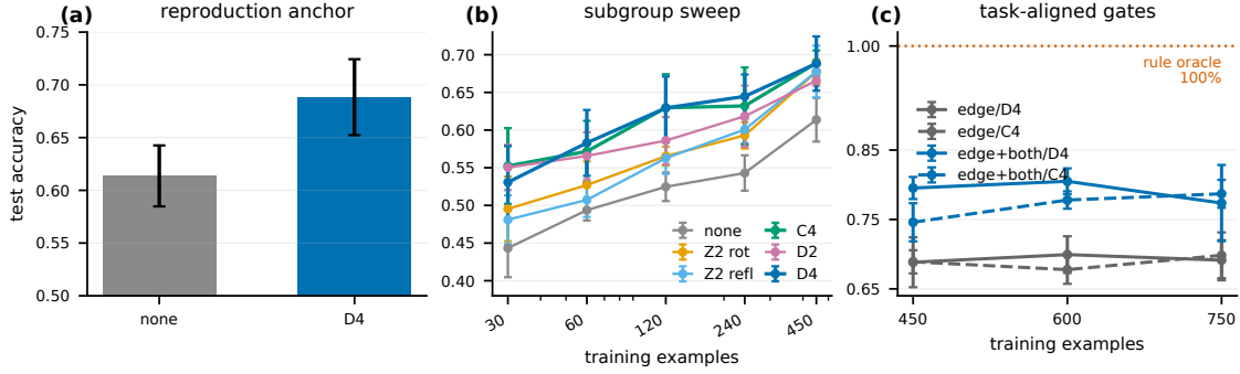
Abbildung 2: Hauptergebnisse. Links: Reproduktion des Meyer-artigen Effekts, D_4 schlägt keine Symmetrie. Mitte: Untergruppen-Sweep über Trainingsgrößen; C_4 folgt D_4 sehr eng. Rechts: Winning-Line-Gates verbessern die Accuracy deutlich, während der deterministische Regel-Oracle als 100%-Referenz dient.
