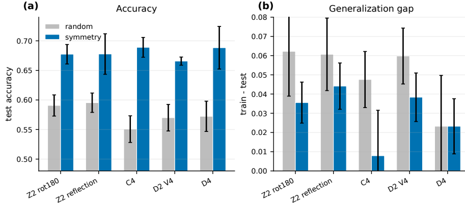
Abbildung 4: Parameter-matched random sharing. Die zufällig geteilten Modelle haben ungefähr dieselbe Parameterzahl wie die jeweiligen Symmetriemodelle, respektieren aber keine Gruppenorbits. Die deutlich schlechtere Test Accuracy zeigt, dass der Effekt nicht bloß eine Folge kleinerer Modelle ist.
