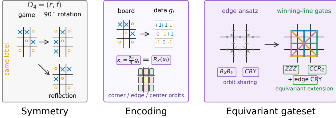
Abbildung 1: Designraum der Arbeit. Ausgehend von der D_4 -Symmetrie des Tic-Tac-Toe-Bretts werden Daten auf neun Qubits kodiert. Untergruppen erzeugen unterschiedliche Parameter-Sharing-Orbits. Die eigene Erweiterung ergänzt den Meyer-artigen Edge-Ansatz um Gates auf den acht Gewinnlinien, ohne die Äquivarianz zu brechen.
