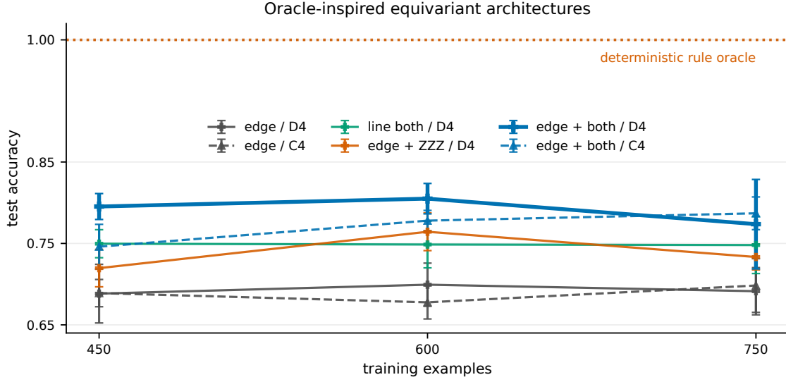
Abbildung 5: Oracle-inspirierte äquivalente Architekturen. Die gestrichelte Linie bei 1.0 ist der deterministische Regel-Oracle und dient nur als obere Referenz. Die beste trainierbare Architektur kombiniert den Edge-Ansatz mit beiden Winning-Line-Kanälen und bleibt D_4 -äquivalent.
