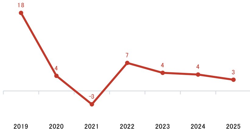
영업이익률 추이 (% , 2019–2025)
