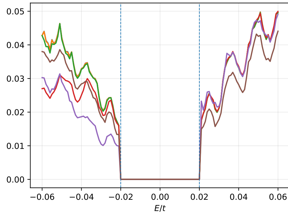
Quasiparticle G_{QP} , 1to2
