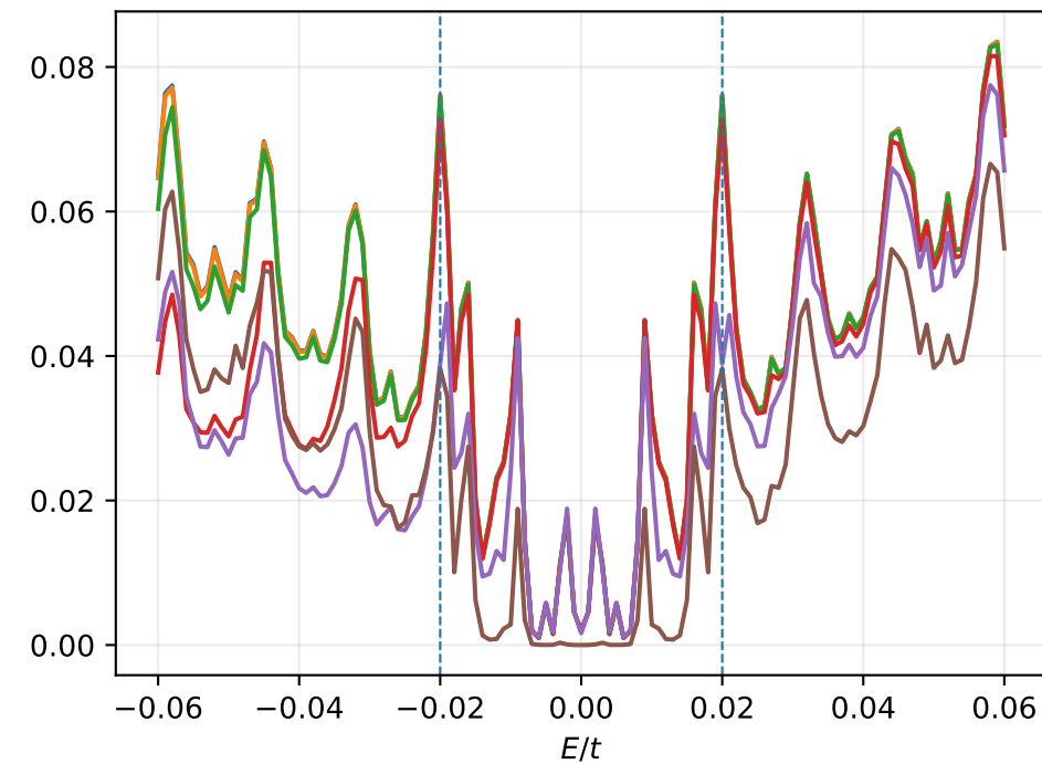
Total G , 1to2
