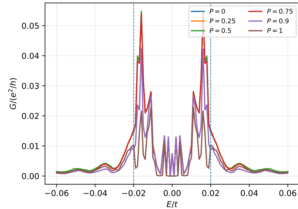
Andreev G_A , 1to2
