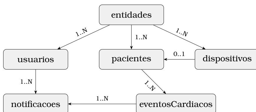
Figura 3.4: Modelo de dados do Firestore : as setas indicam as referências entre coleções e a respectiva cardinalidade.
