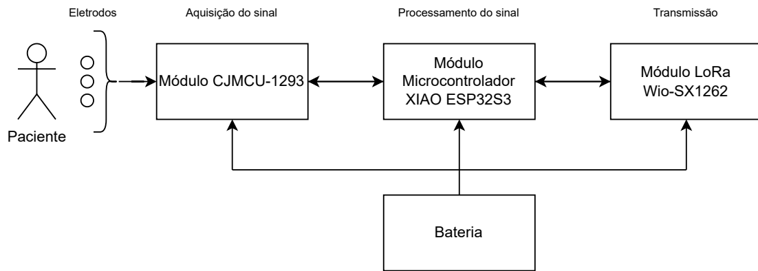
Figura 3.2: Diagrama de blocos do dispositivo de aquisição e transmissão do sinal de ECG.
