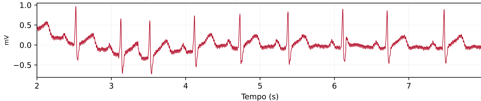
Sinal FILTRADO — filtro IIR aplicado em software (réplica do firmware) (LeadII)
