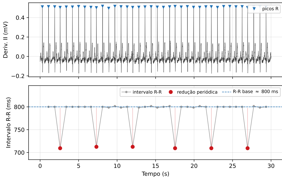
Figura 4.5: Perda de amostras no sinal bruto de um segmento normal (75 bpm) indevidamente classificado como arritmia. Acima, a derivação II adquirida, com os picos R detectados; abaixo, a série de intervalos R-R, na qual se observam seis reduções periódicas — de \approx 800 para \approx 710 ms, a cada \approx 4,9 s —, coincidentes com o bloqueio do laço de aquisição pela rotina de diagnóstico.
