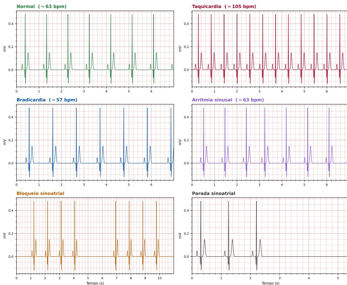
Figura 4.6: Exemplos das seis classes de estímulo empregadas na validação final, reproduzidos pelo gerador NI myDAQ e apresentados na escala de amplitude medida na entrada do AFE. No painel de bloqueio a janela é centrada na pausa — de 3,00 vezes o intervalo R-R mediano, equivalente à ausência de dois complexos QRS —, de modo que se observe a retomada do ritmo; no de parada, a janela mostra primeiro os batimentos e termina dentro da pausa, de 3,50 vezes o intervalo mediano.
