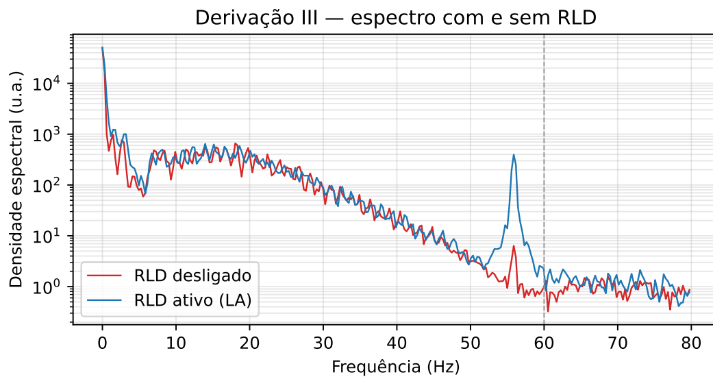
Figura 4.3: Espectro da derivação III no teste de bancada, com o RLD desconectado e ativo. A linha tracejada indica a frequência da rede elétrica (60 Hz).
