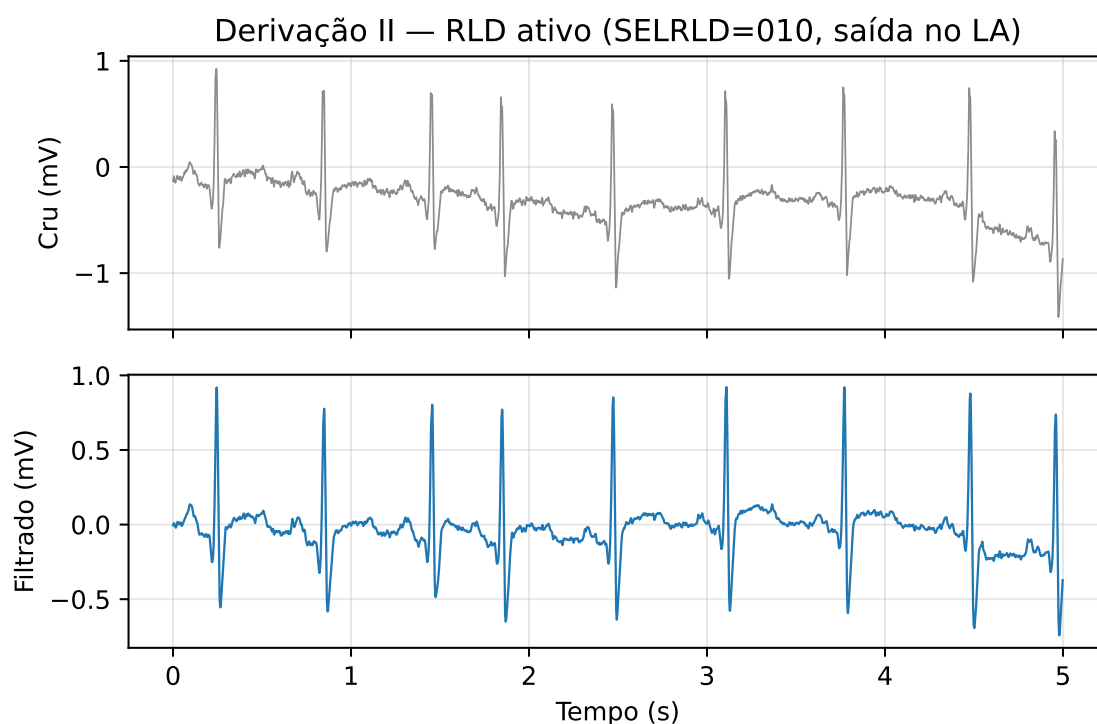
Figura 4.1: Trecho de 5 s da derivação II adquirida no teste de bancada, com o RLD ativo: sinal bruto (acima) e após a cadeia de filtros digitais do firmware (abaixo).
