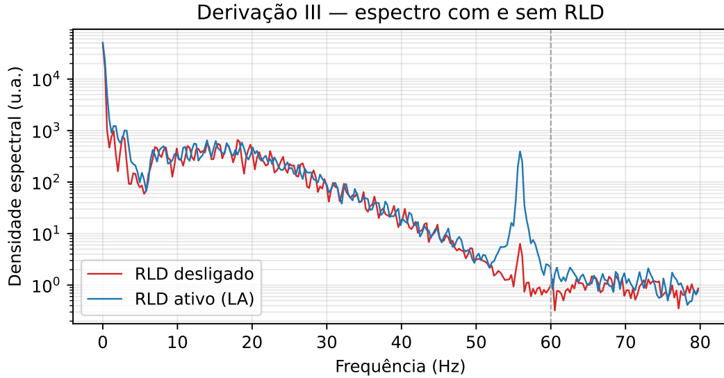
Figura 4.2: Espectro da derivação III no teste de bancada, com o RLD desconnectado e ativo. A linha tracejada indica a frequência da rede elétrica (60 Hz).
