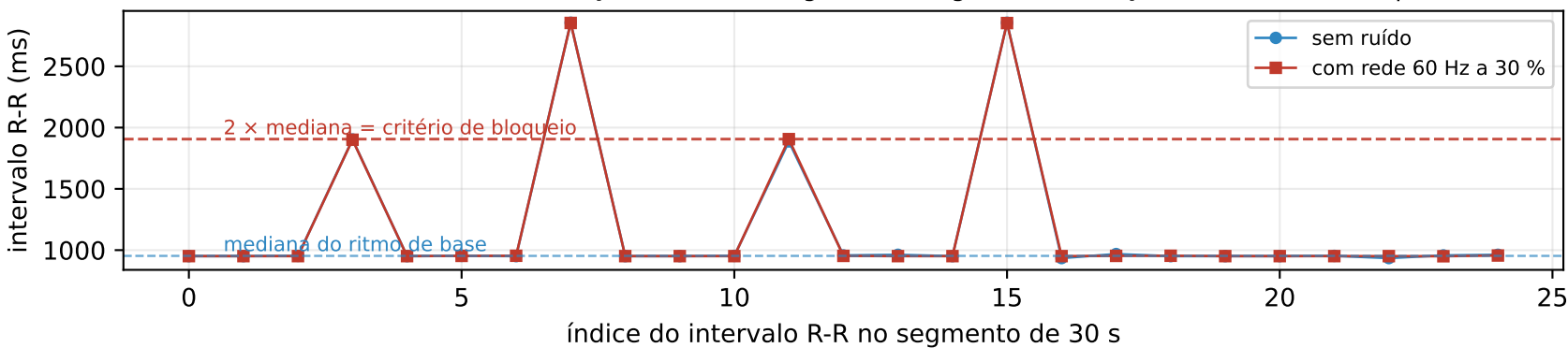
(d) Intervalos R-R em SIMULAÇÃO — o ruído digital não degrada a detecção (classificado: bloqueio)
