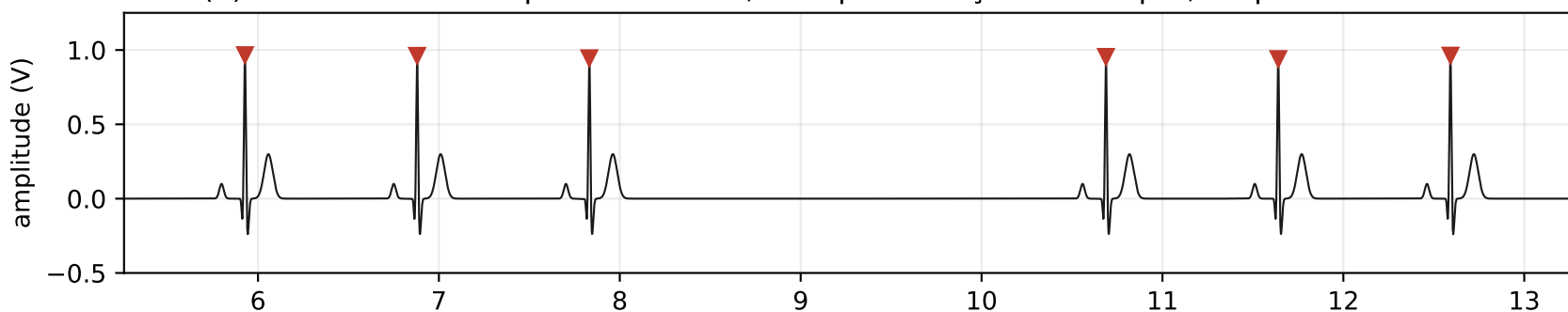
(a) Estímulo com bloqueio sinoatrial, sem perturbação — 50 bpm, 26 picos R em 30 s
