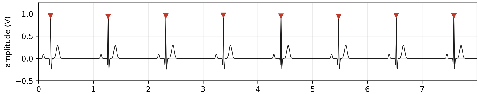
(a) Estímulo com bradicardia, sem perturbação — 57 bpm, 29 picos R em 30 s
