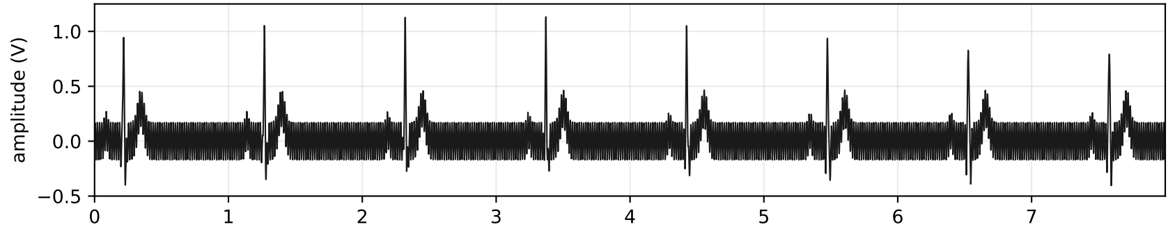
(b) Com interferência de rede de 60 Hz a 30 % — 57 bpm, 29 picos R em 30 s
