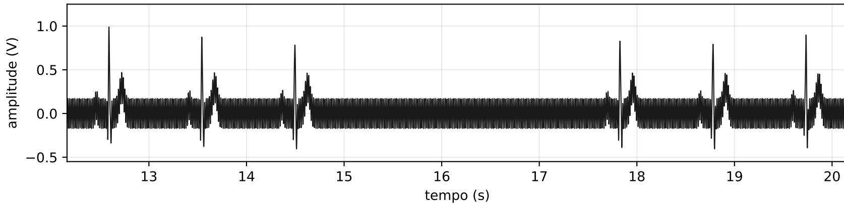
(b) Com interferência de rede de 60 Hz a 30 % da excursão
