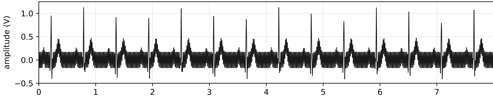
(b) Com interferência de rede de 60 Hz a 30 % — 84 bpm, 43 picos R em 30 s
