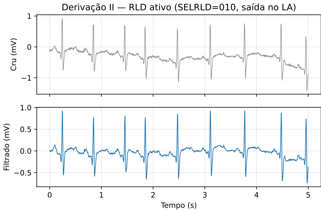
Figura 4.2: Trecho de 5 s da derivação II adquirida no teste de bancada, com o RLD ativo: sinal bruto (acima) e após a cadeia de filtros digitais do firmware (abaixo).
