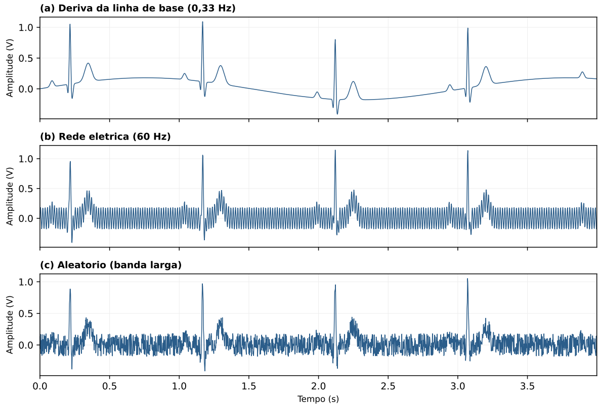
Figura 4.8: Estímulo normal com cada um dos três tipos de ruído somado a 30% da excursão do sinal: (a) deriva da linha de base a 0,33 Hz; (b) interferência de rede a 60 Hz; (c) ruído aleatório de banda larga. Trecho de 4 s.
