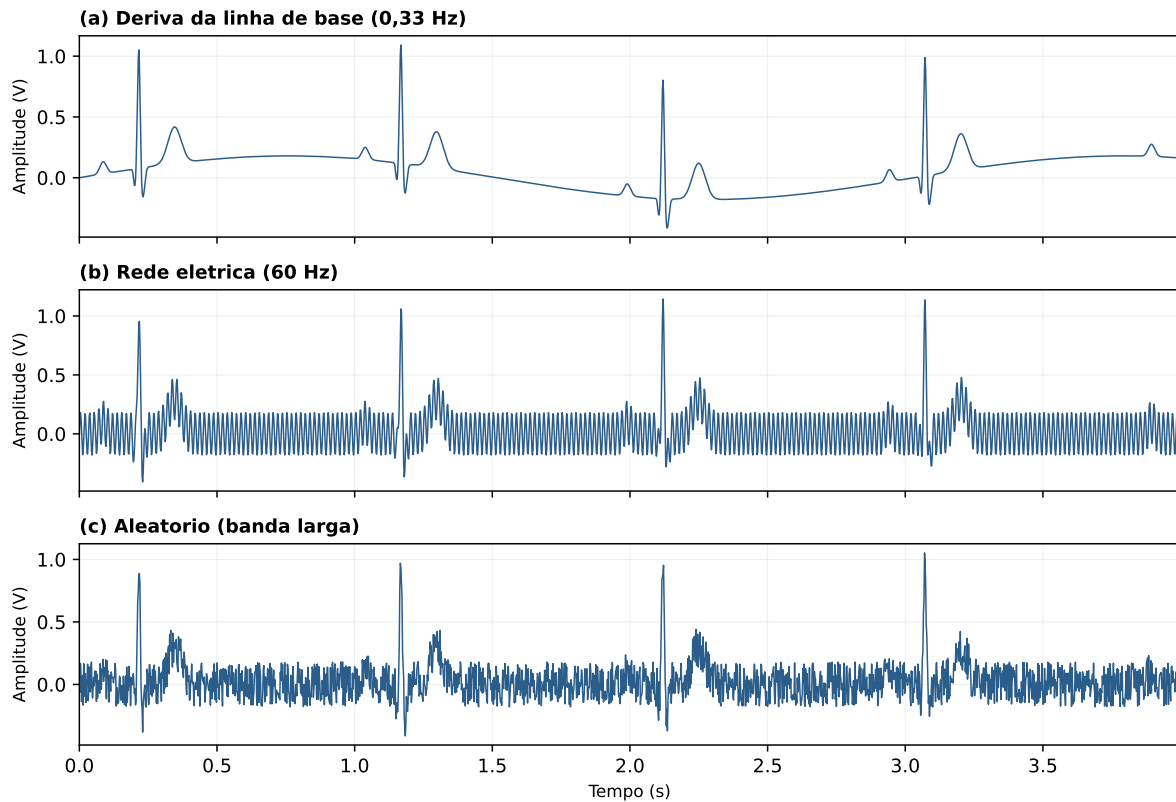
Figura 4.6: Estímulo normal com cada um dos três tipos de ruído somado a 30 % da excursão do sinal: (a) deriva da linha de base a 0,33 Hz; (b) interferência de rede a 60 Hz; (c) ruído aleatório de banda larga. Trecho de 4 s.
