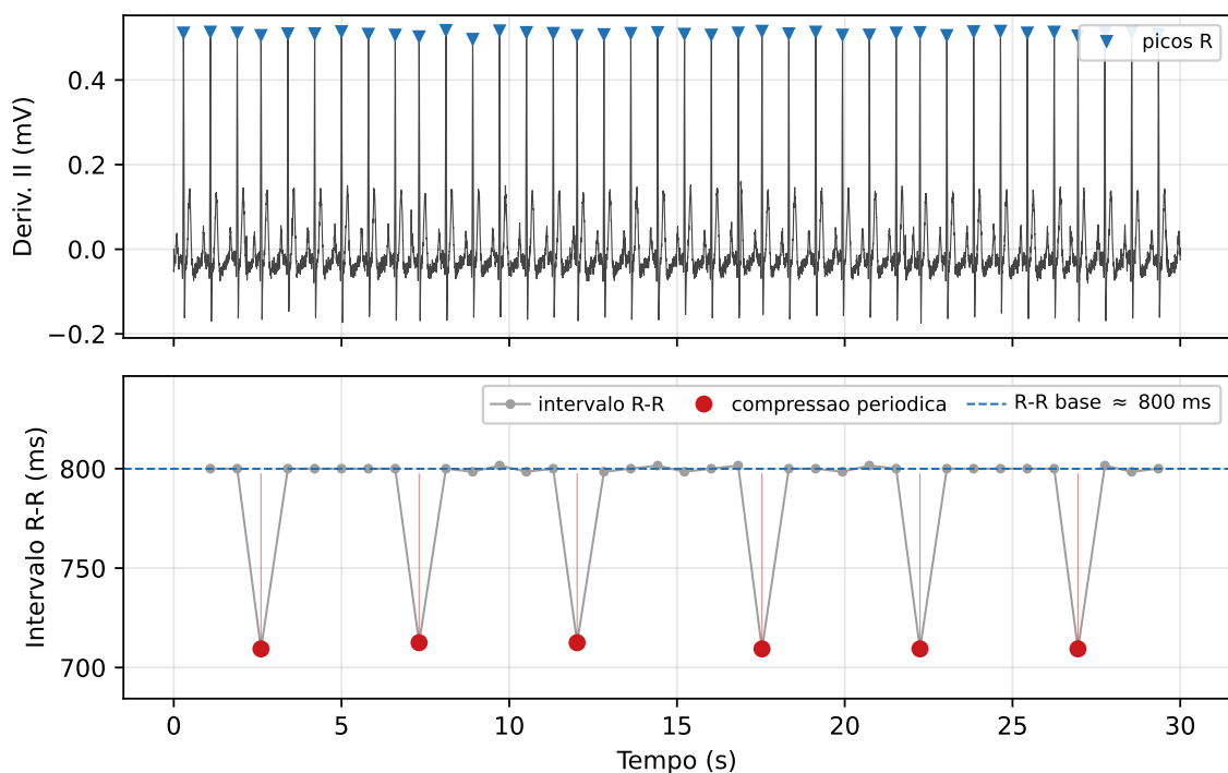
Figura 4.4: Artefato de perda de amostras no sinal bruto de um segmento normal (75 bpm) indevidamente classificado como arritmia. Acima, a derivação II adquirida, com os picos R detectados; abaixo, a série de intervalos R-R, na qual se observam seis compressões periódicas — de \approx 800 para \approx 710 ms, a cada \approx 4,9 s —, coincidentes com o bloqueio do laço de aquisição pela rotina de diagnóstico. As quedas aproximam a diferença entre intervalos sucessivos do limiar de arritmia (120 ms), produzindo a detecção indevida.
