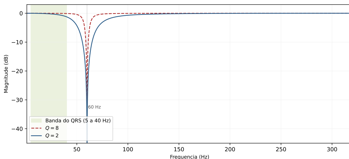
Figura 4.7: Resposta em frequência do filtro notch de 60 Hz para os dois fatores de qualidade avaliados ( Q = 8 e Q = 2 ), à taxa de amostragem de 640 SPS. Ambos anulam a componente de 60 Hz; o filtro mais largo ( Q = 2 ) atenua levemente a borda superior da banda do QRS, mas reduz a duração da resposta transitória responsável pela introdução de picos indesejados.
