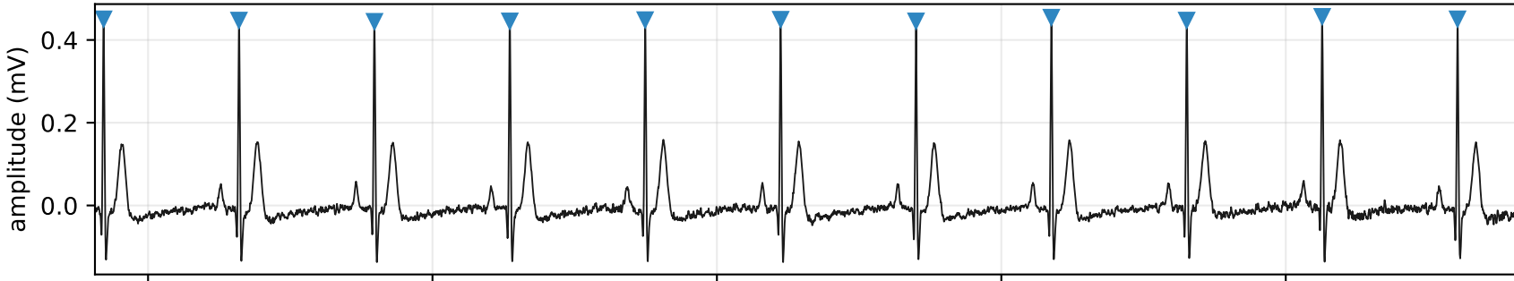
Sem perturbação — 11 QRS no sinal, 11 detectados
