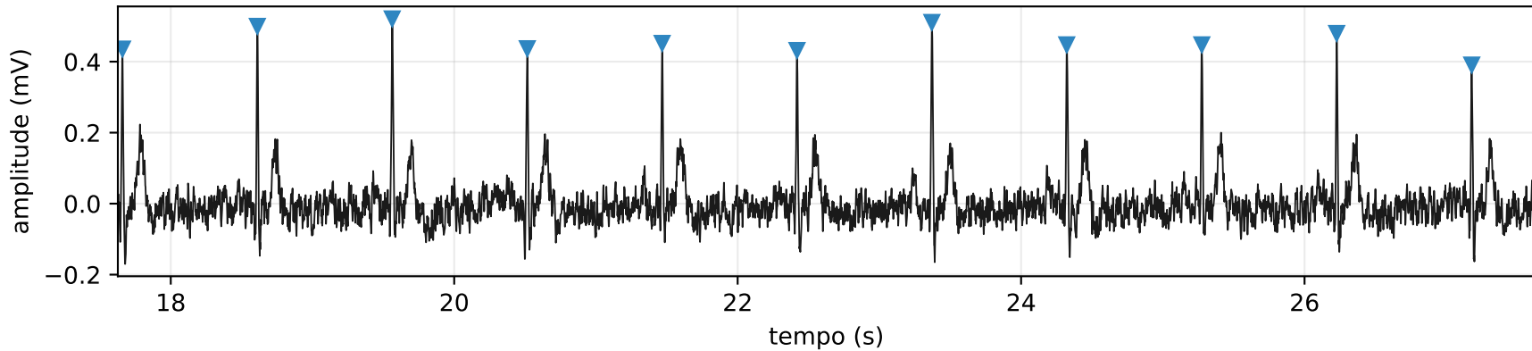
Aleatório a 30 % — 11 QRS no sinal, 11 detectados
