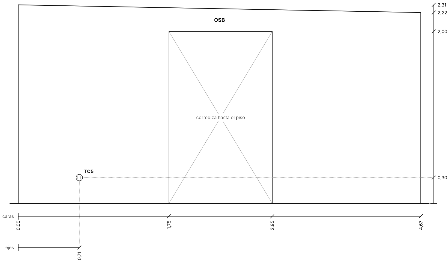
MURO D Vista desde el interior
