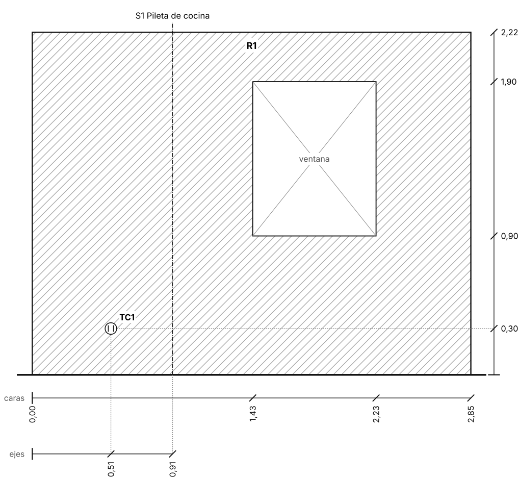
MURO A Vista desde el interior
