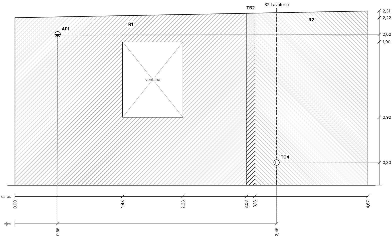
MURO B Vista desde el interior
