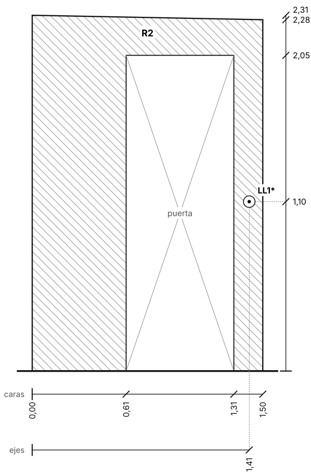
TABIQUE TB3 · CARA HACIA B Vista desde el interior
