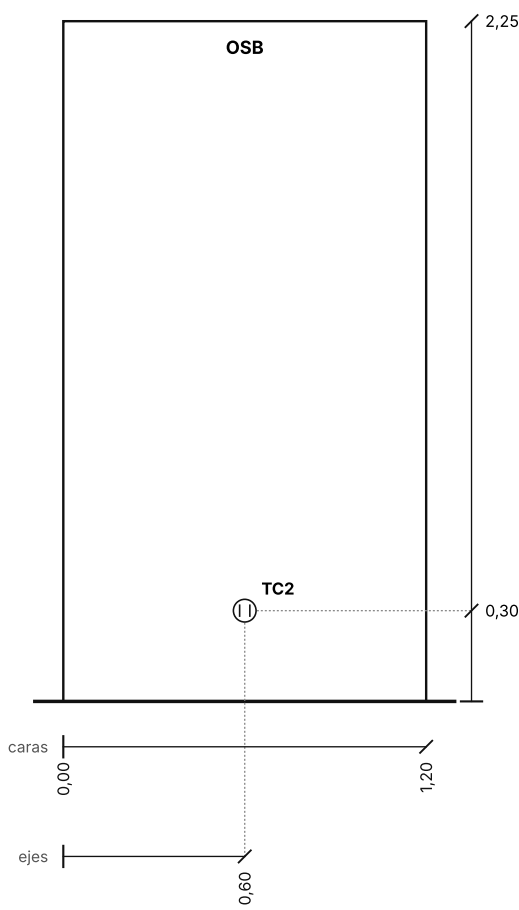
TABIQUE TB1 · CARA HACIA A Vista desde el interior
