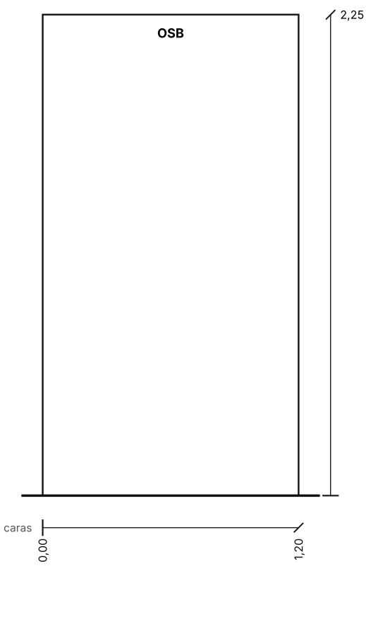
TABIQUE TB1 · CARA HACIA C Vista desde el interior
