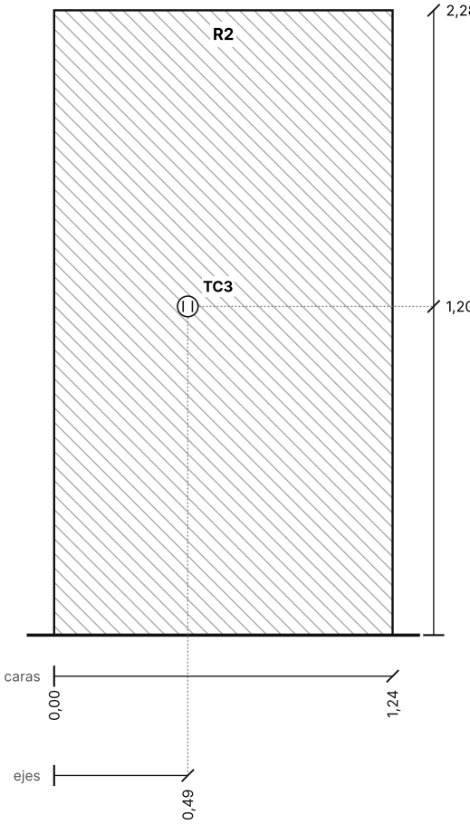
TABIQUE TB2 · CARA HACIA C Vista desde el interior
