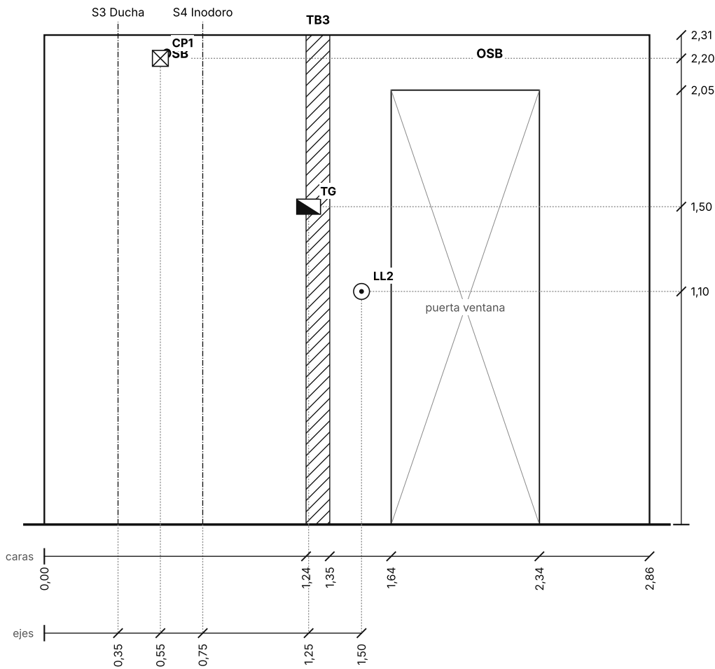
MURO C Vista desde el interior
