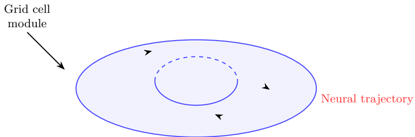
(D) Grid Cell Population Activity on T^2
