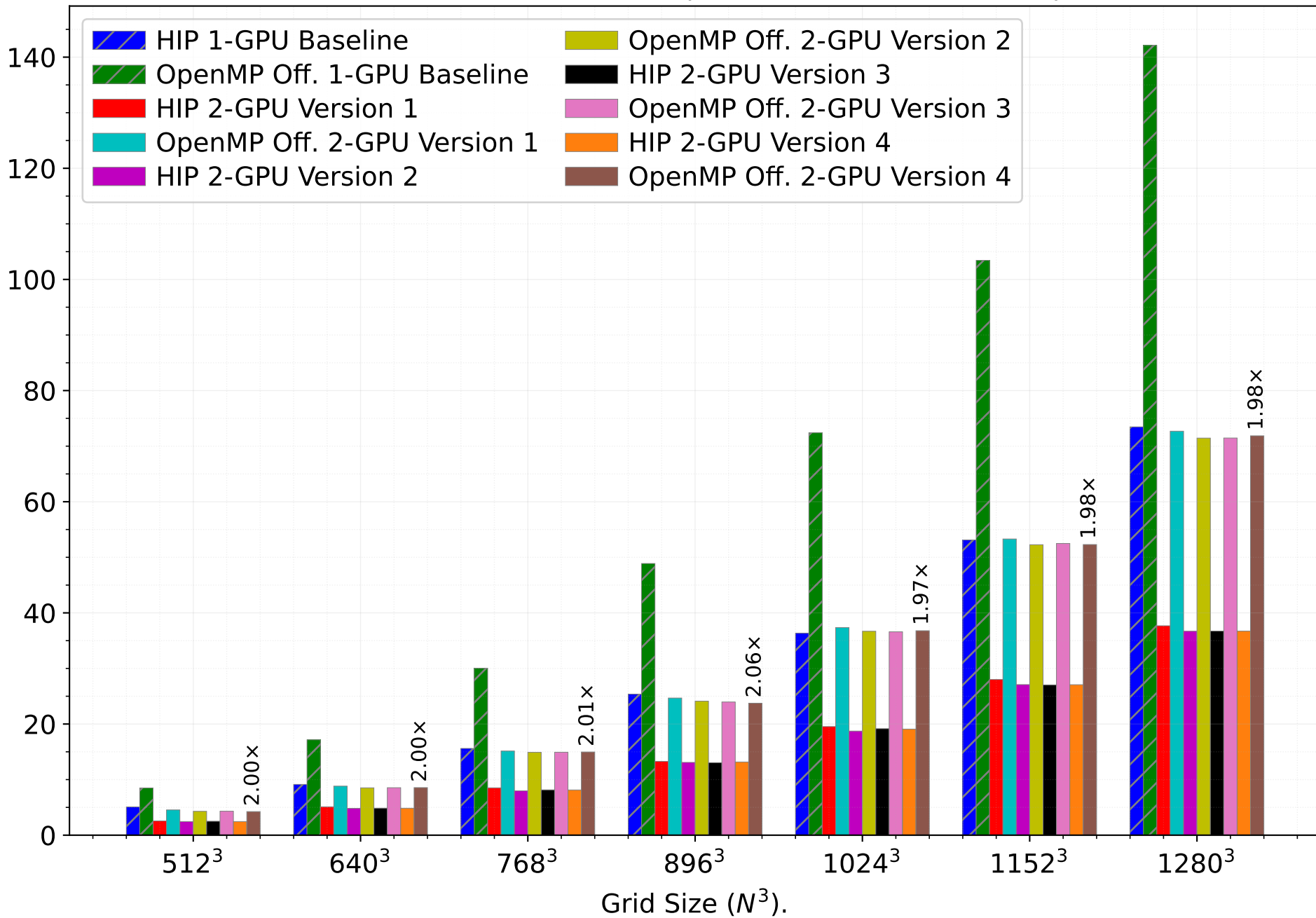
AMD MI250X - 2 GPUs (1 GCD per module) (~500 time steps).
