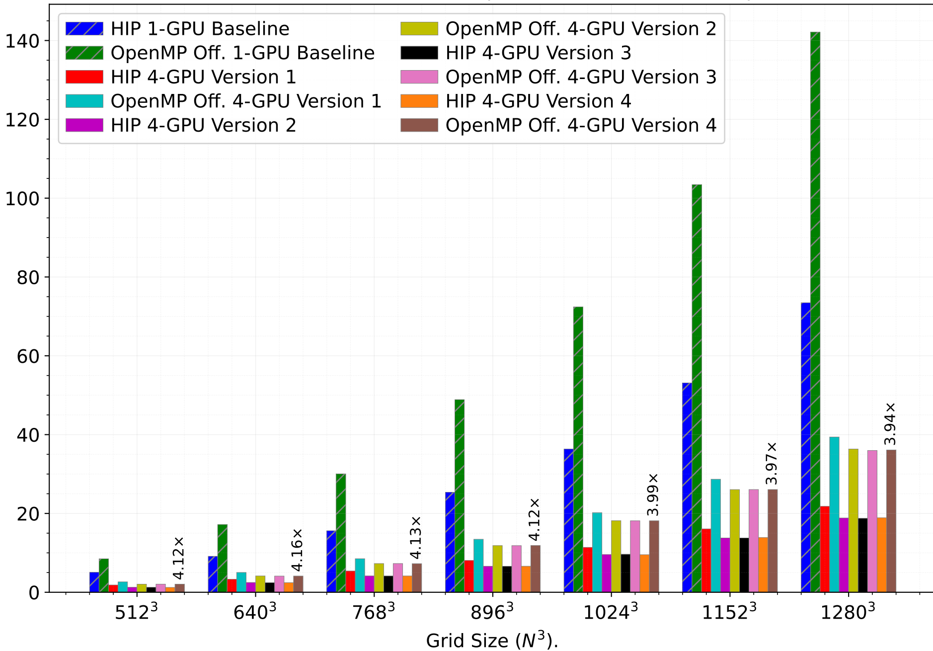
AMD MI250X - 4 GPUs (1 GCD per module) (~500 time steps).
