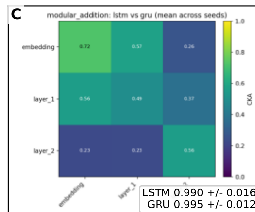
LSTM vs GRU
