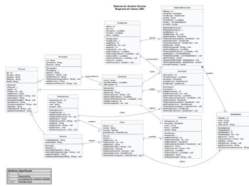
Diagrama de Clases UML - SGE
