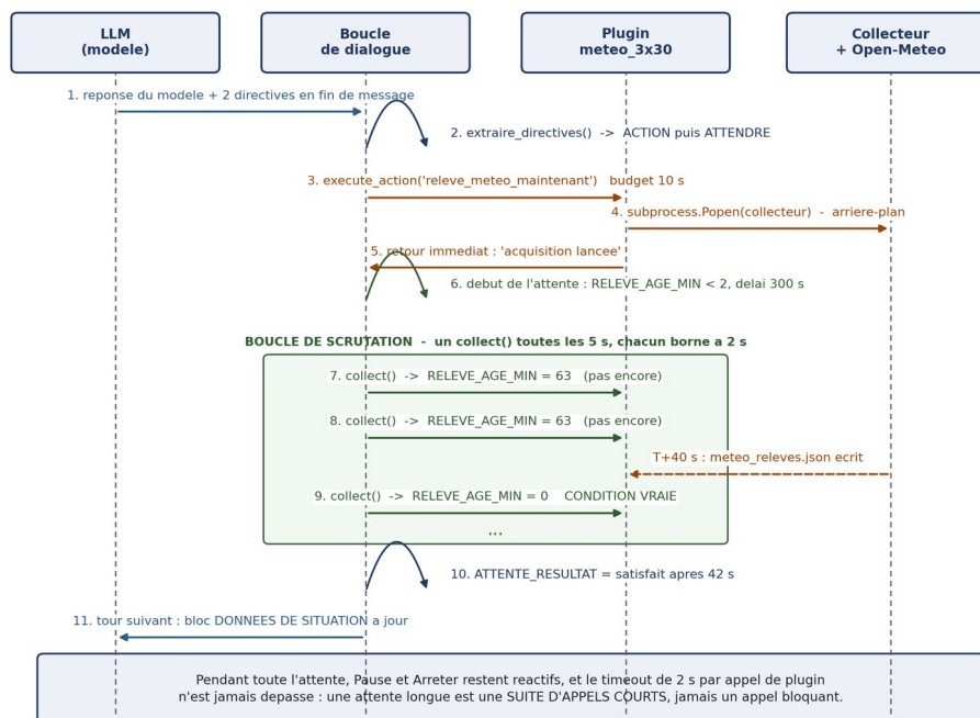
Figure 3 — Séquence d'une action suivie d'une attente
