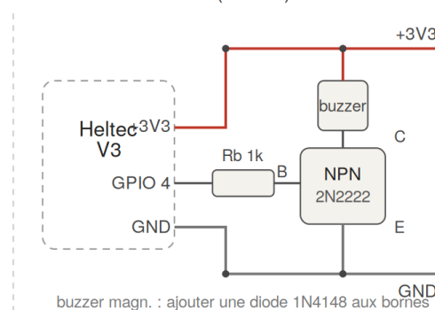
Figure 2 — Câblage du buzzer sur GPIO : piezo direct (A) ou via transistor (B).
