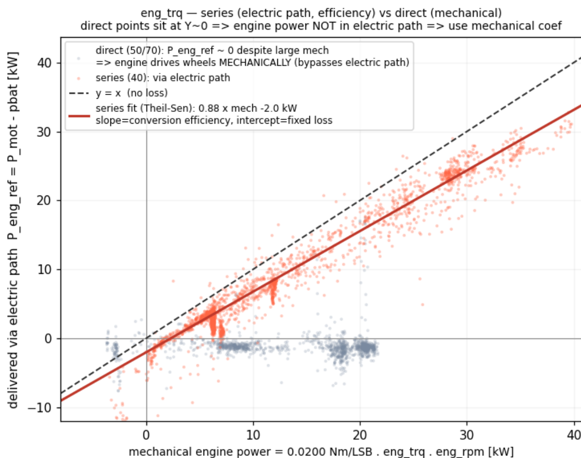
Fig7. エンジン出力の較正と効率。 シリーズで届いたエンジン出力 P_{eng\_ref} を機械出力に Theil-Sen で回帰し、傾き 0.88 (効率) を得た。灰色点は直結で P_{eng\_ref} \approx 0 となり、機械直結経路であることを示す。
