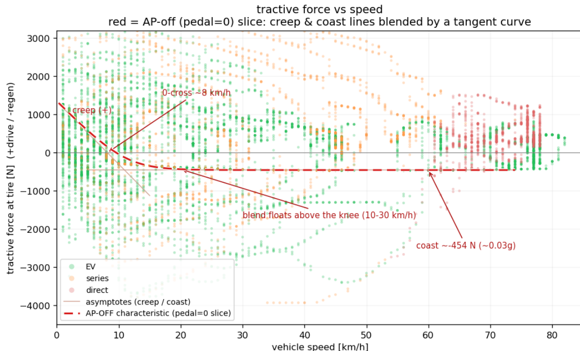
Fig13. 踏面駆動力（モード別）と AP OFF 特性ライン。同定トルクから式 (5)-(7) で再構成した踏面駆動力。赤破線はアクセル 0 固定・車速スweepの支配ライン（クリープ → コースト回生）。
