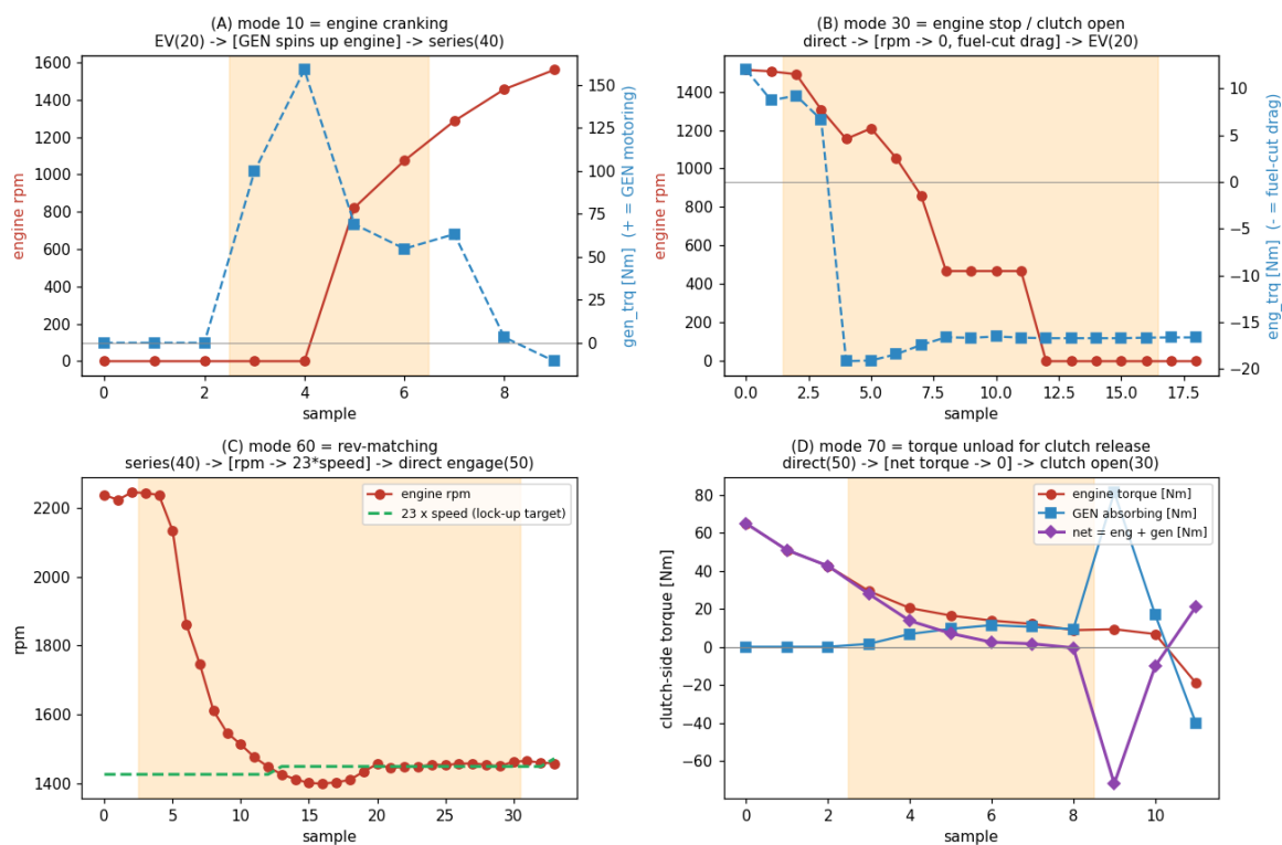
Fig9. 過渡モードの時系列。A: 始動クランキング (10)、B: 停止・クラッチ開放 (30)、C: レブマッチ係合 (60)、D: トルクアンロード (70)。各部トルク・rpm の挙動が各機序を裏付ける。
