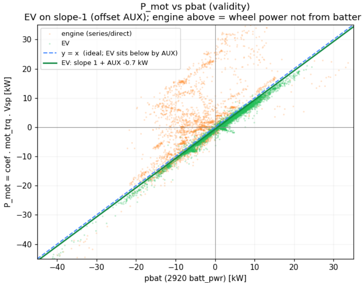
Fig6. 再構成した P\_mot と実測 pbat の比較。EV（緑）は傾き 1 + AUX で一致し、エンジン時（橙）は電池を介さない駆動分だけ上へ乖離する。
