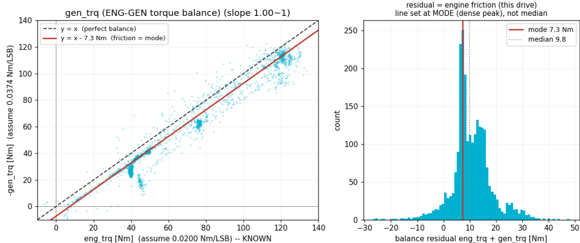
Fig8. 発電機トルクの釣り合い（シリーズ）。 -\text{gen\_trq} [Nm] と \text{eng\_trq} [Nm] が傾き 1.00 で釣り合う。切片 \approx 7.3\text{Nm} がエンジン内部フリクションに相当する。
