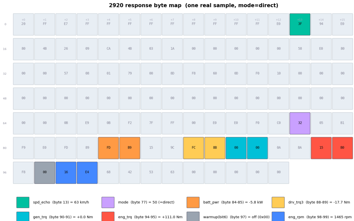
Fig12. 2920 応答のバイトマップ (直結時 1 サンプル)。 生 HEX に同定フィールドを重ね、バイト範囲と物理値の対応を示す。
