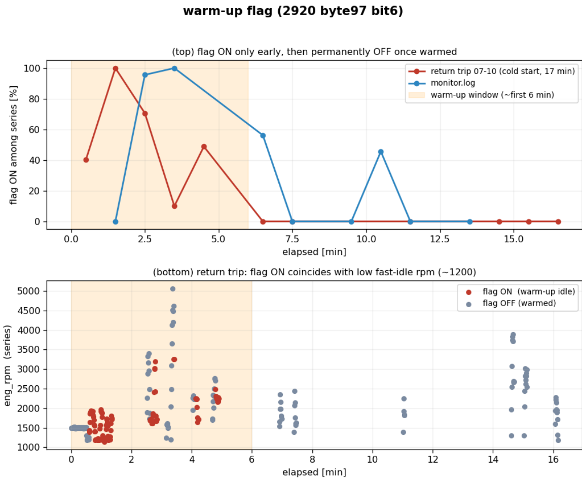
Fig10. 暖機フラグの時間挙動。 上：フラグは冷間序盤 ~6 分のみ ON し、以降 OFF を保つ。下：ON 区間でエンジンは低回転ファストアイドル (~1200rpm) に居る。
