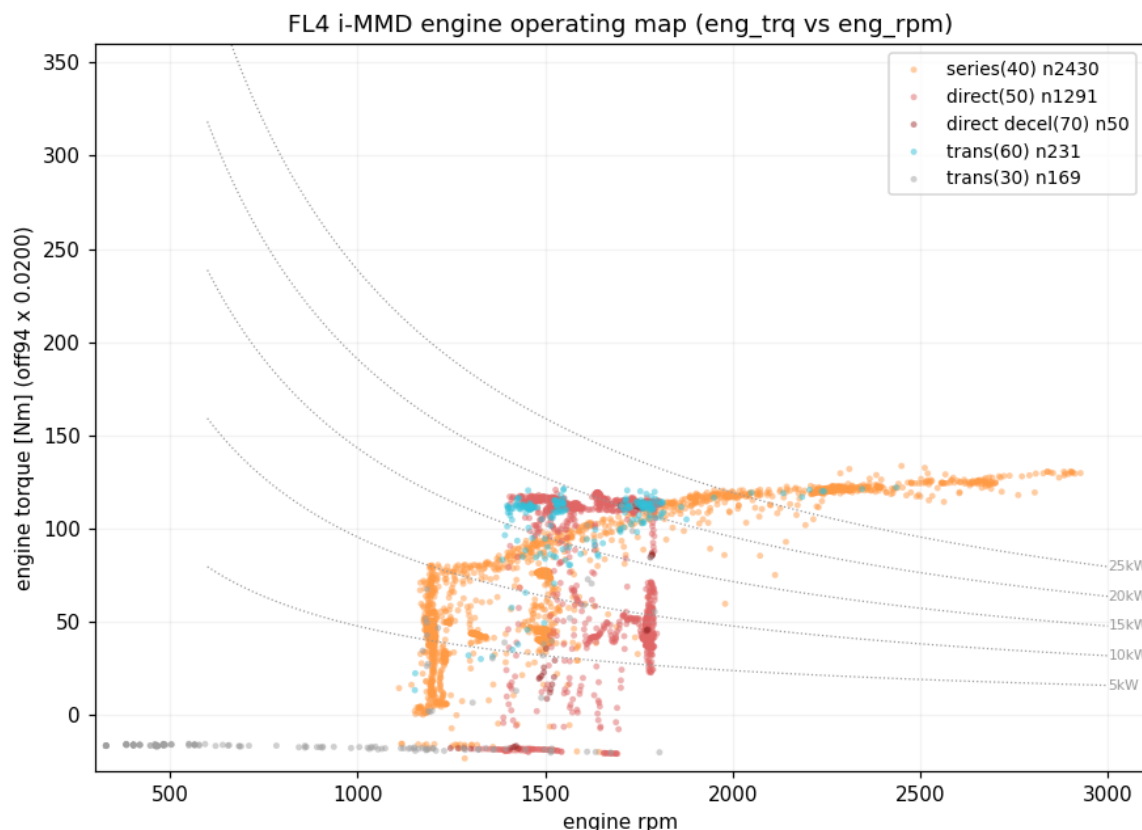
Fig11. エンジン動作マップ。シリーズ（橙）は効率最適の運転ラインを成し、直結（赤）は車速で rpm が拘束されトルクが縦に散る。下端はフューエルカット時のドラッグトルク。
