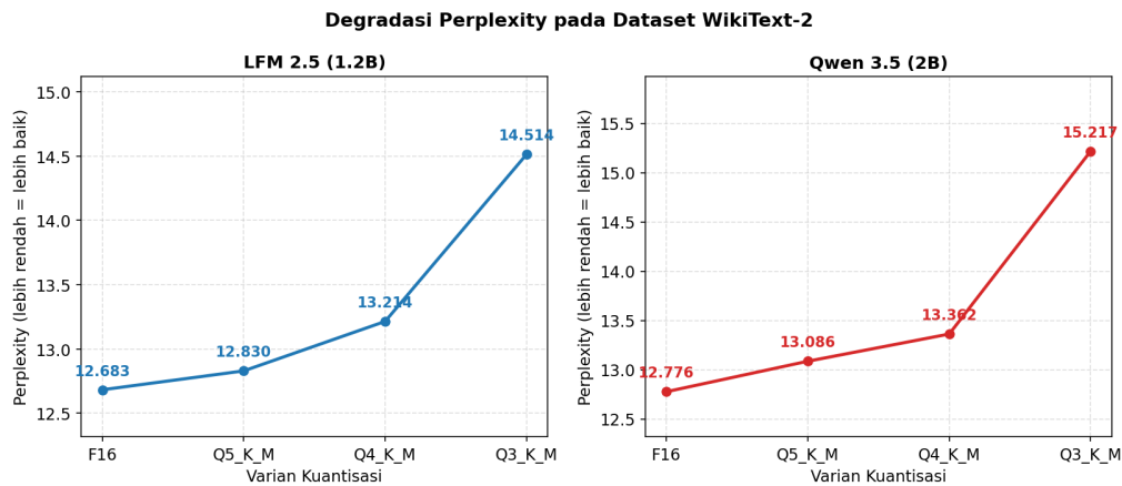
Gambar 4.4 Degradasi Perplexity pada dataset WikiText-2. Sumber: olahan penulis.
