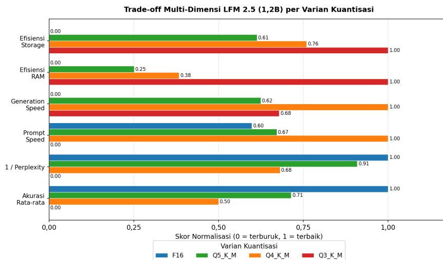
Gambar 4.6 Diagram trade-off multi-dimensi LFM 2.5 (1,2B) per varian kuantisasi (skor normalisasi 0..1, lebih tinggi = lebih baik). Sumber: olahan penulis.
