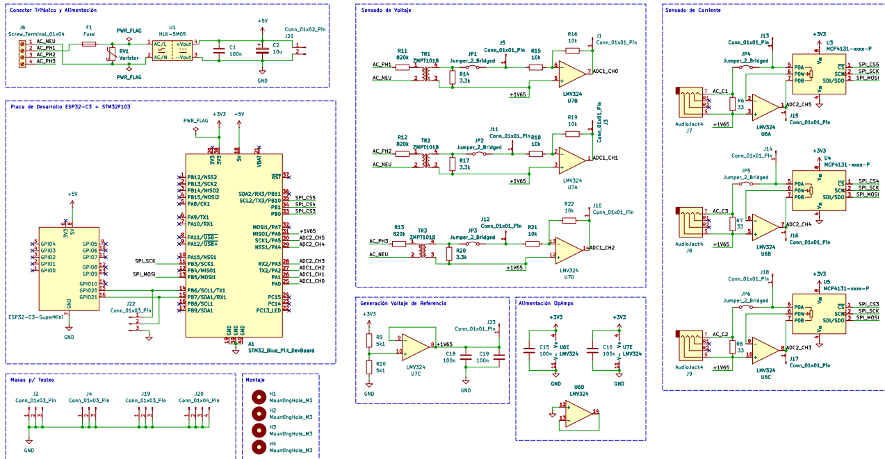
Figura 2: Diagrama esquemático general del sistema de medición y gateway.
