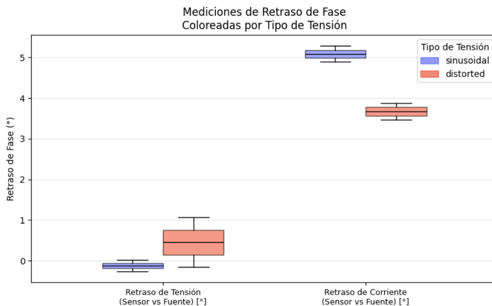
Figura 6: Diagrama de caja del desfase medido, agrupado por tipo de señal de tensión.
