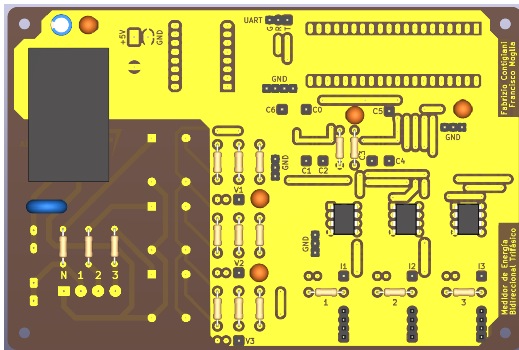
Figura 15: Renderizado 3D detallado de la placa ensamblada.
