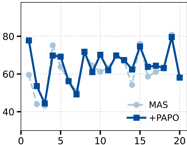
TRGP
