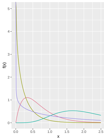
Gamma Verteilung
