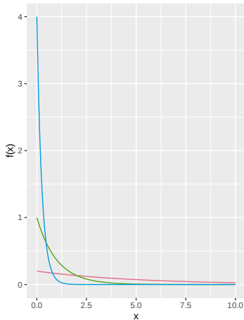
Exponential Verteilung
