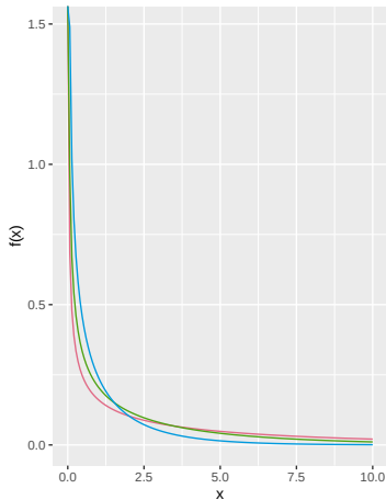
Gamma Verteilung
