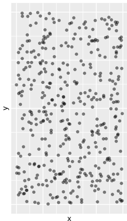
Gesamtbevölkerung
