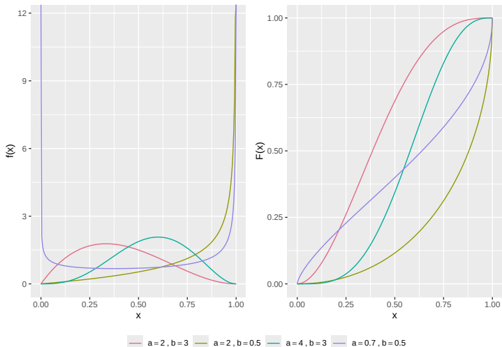
Beta-Verteilung
