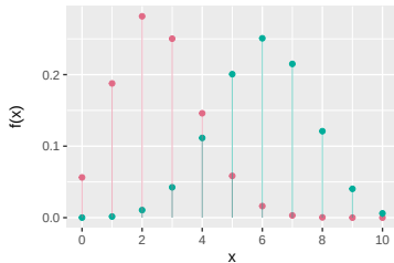
Binomial Verteilung
