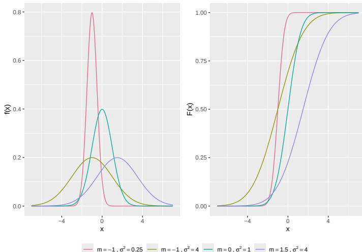
Normal-Verteilung
