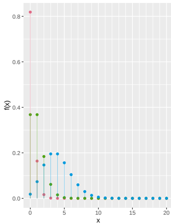
Poisson Verteilung
