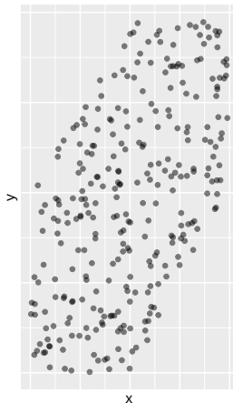
Beobachtet falls |x - y| < \text{const}
