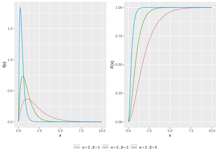
Gamma Verteilung
