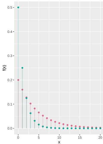
Geometrische Verteilung
