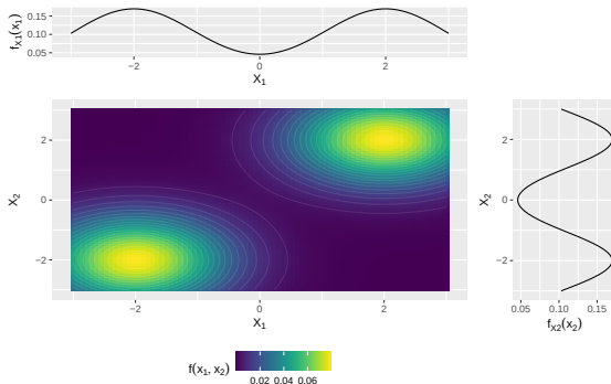
Abhängige Zufallsvariablen
