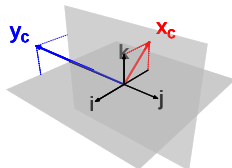
zentrierte Datenvektoren
